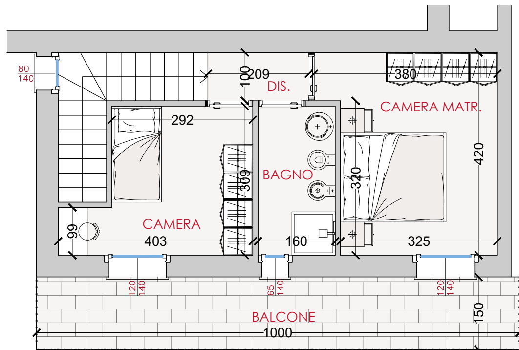
Piano secondo
