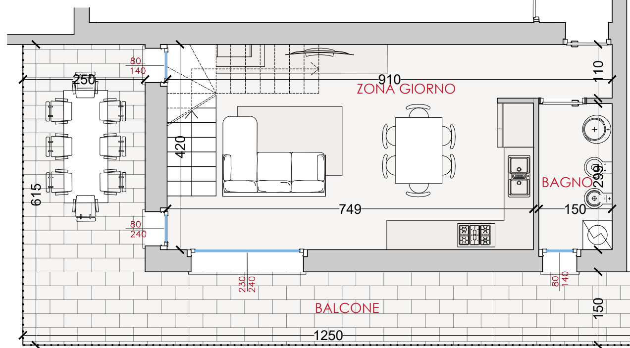
Piano primo
