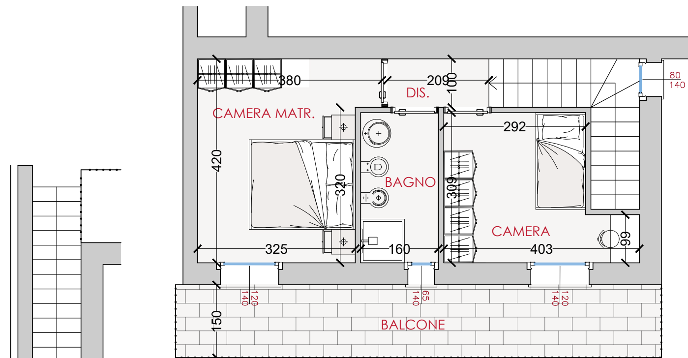
Piano secondo
