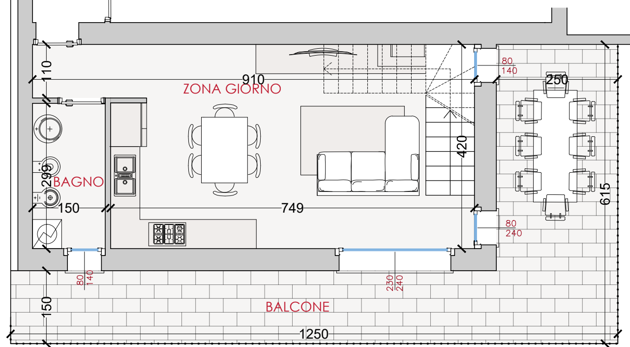
Piano primo
