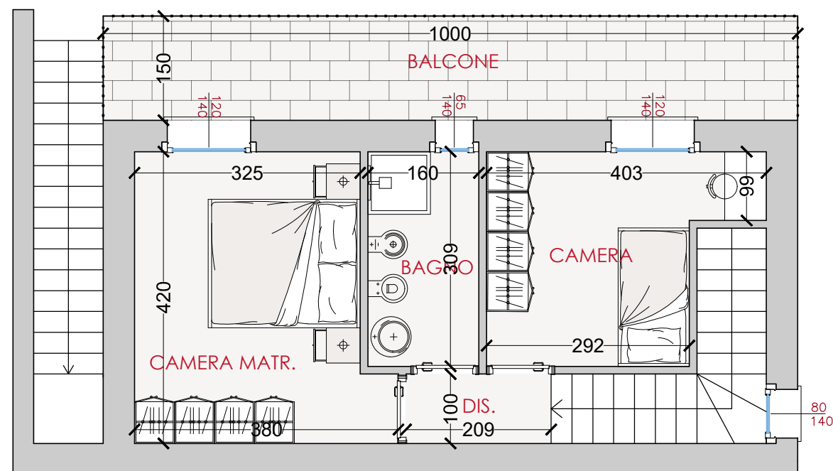
Piano secondo
