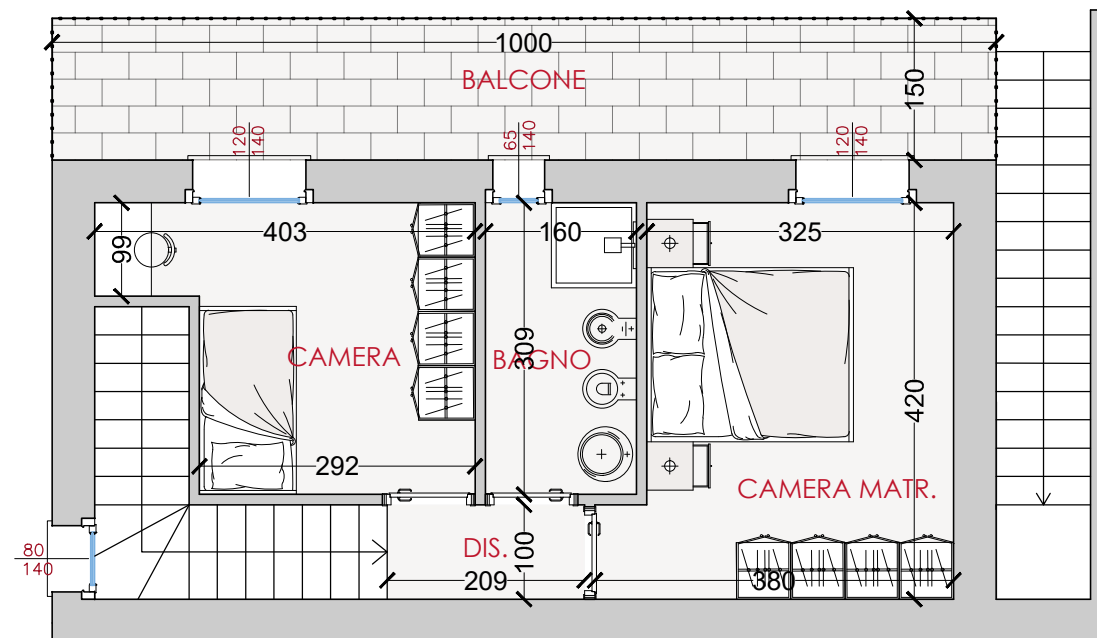
Piano secondo
