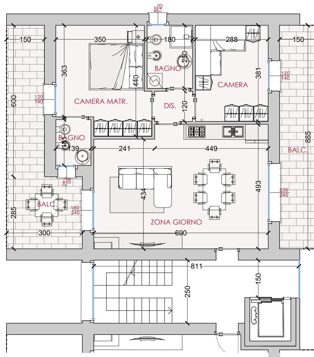
Piano primo
